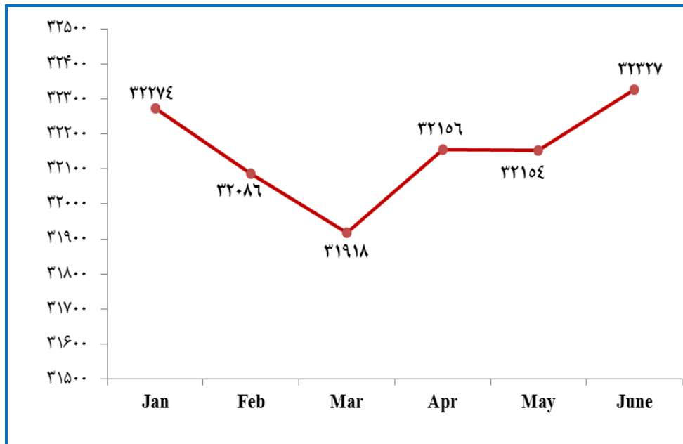
تولید نفت خام ماهانه اوپک (هزار بشکه در روز)، Jan- June 2018
