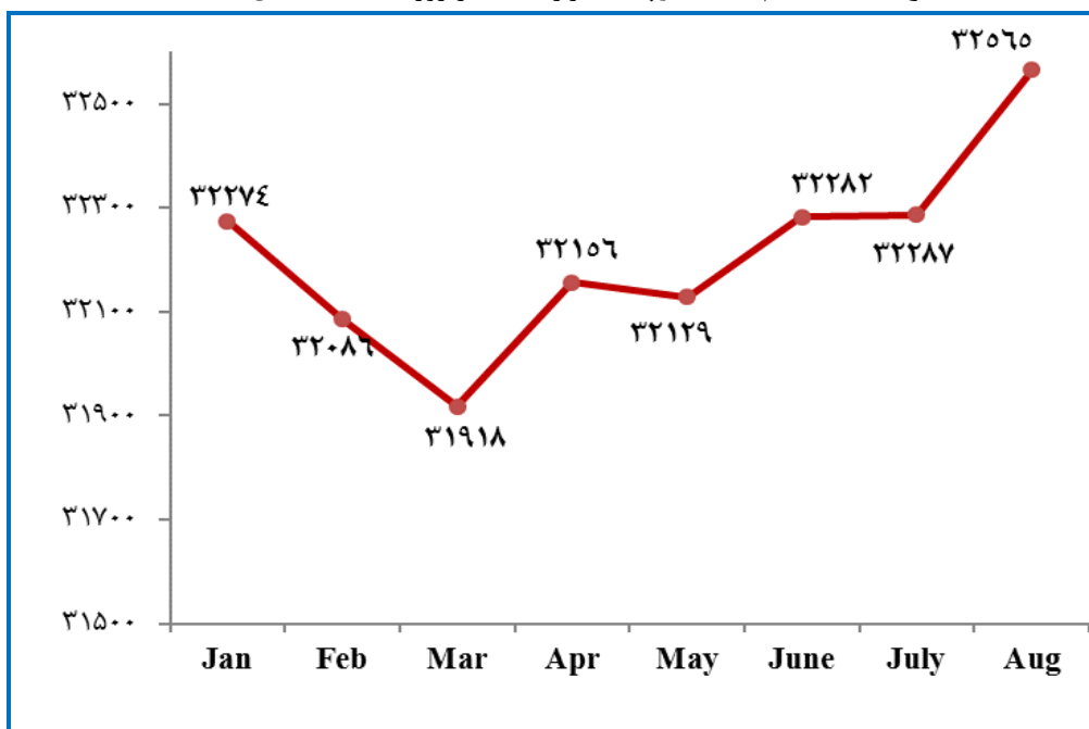
تولید نفت خام ماهانه اوپک (هزار بشکه در روز)، ۸ ماهه سال ۲۰۱۸
